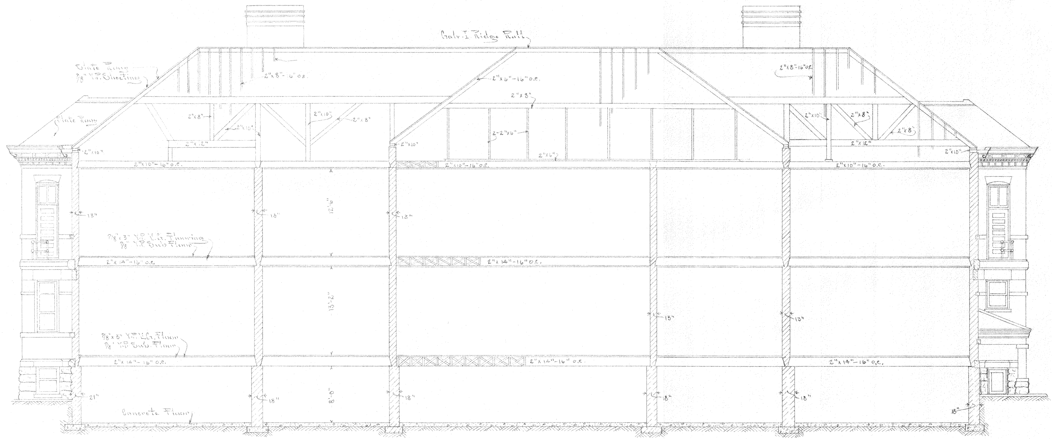
LONGITUDINAL - SECTION
